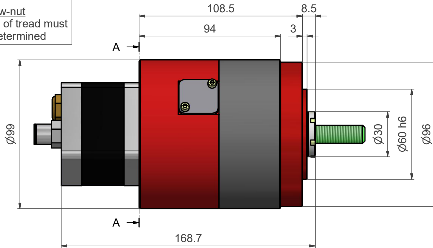
Schnitt A-A (1 : 1.5)
