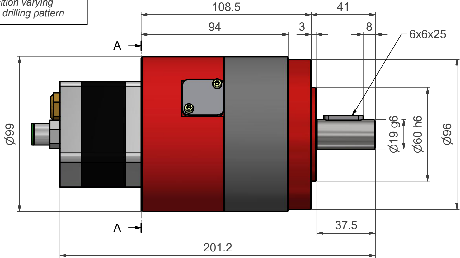
Schnitt A-A (1 : 1.5)
